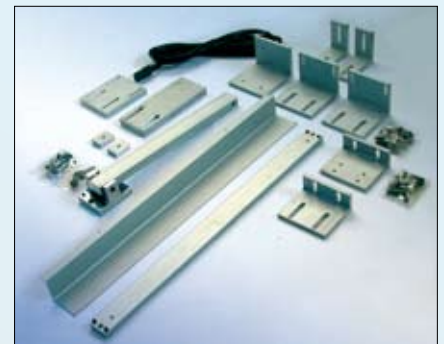
Een complete montageset met draagarm, aanbouwprofielen en -platen, enz. behoort tot het standaardtoebehoren.
