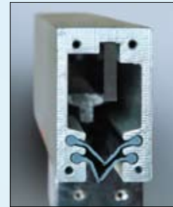
Een robuuste aluminiumkast met dubbele afdichtlippen beschermt glasliniaal en aftastunit tegen spaanders, stof en spatwater.
